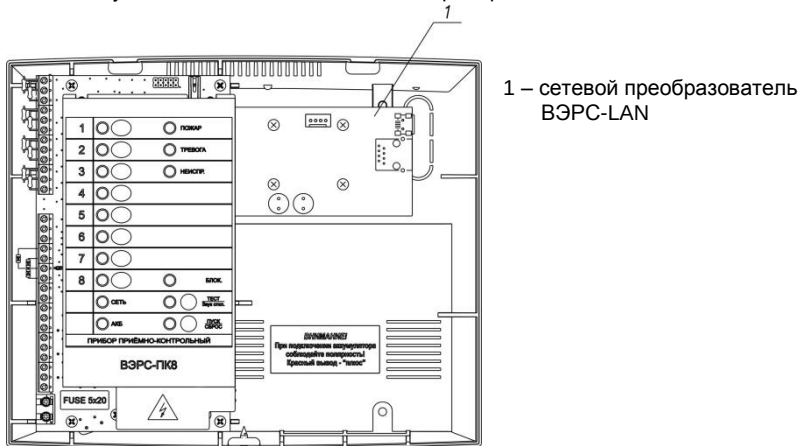
Рисунок Б3. Внешний вид сетевого преобразователя ВЭРС-LAN.
