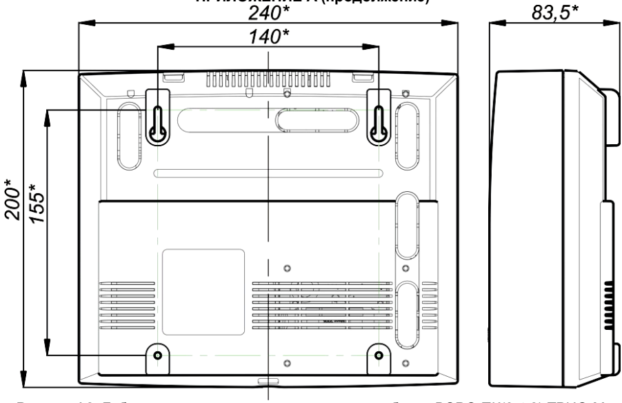
Рисунок А2. Габаритные и установочные размеры приборов ВЭРС-ПК(8,4,2) ТРИО-М.
