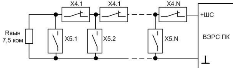
Рисунок Б5. Схема включения линейных дымовых извещателей ИПДЛ-Д-II/4P.
