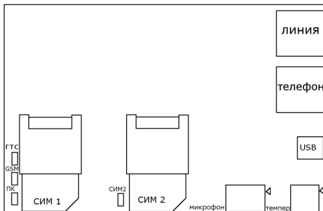
Рисунок Б9. Вид на индикаторы и разъемы модуля МАД.
