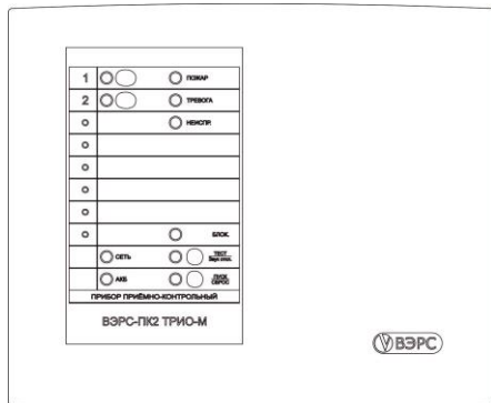
а) ВЭРС-ПК2 ТРИО-М
