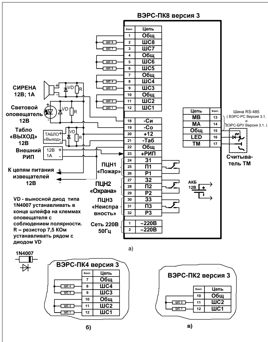
Рисунок.Б1. Схемы внешних соединений приборов ВЭРС-ПК(8,4,2) ТРИО-М.
