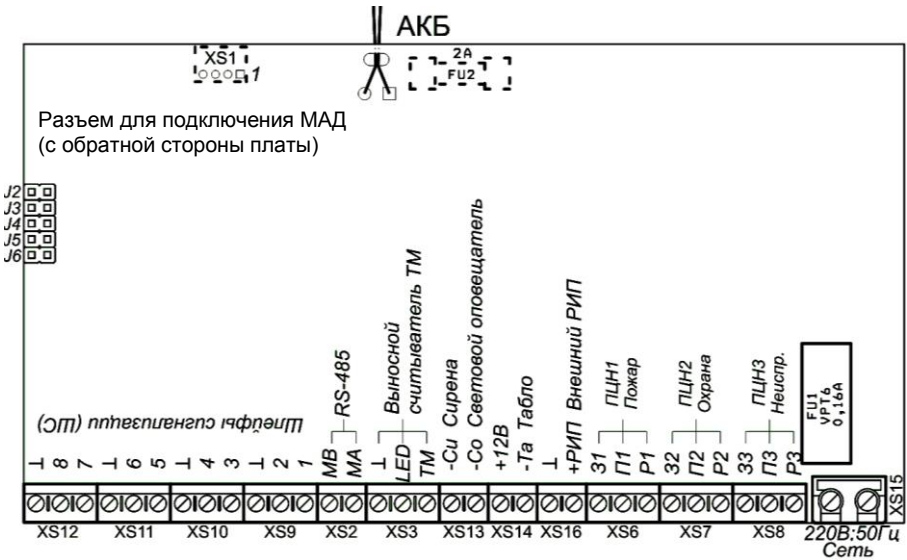
Рисунок А3. Вид на клеммы и разъемы для внешних подключений ВЭРС-ПК(8,4,2) ТРИО-М
