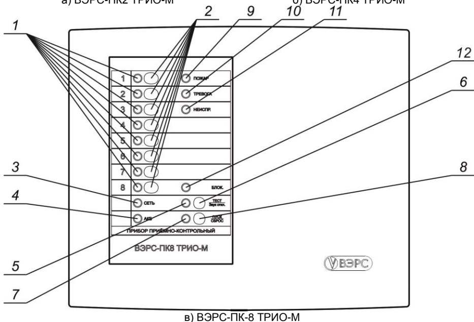
в) ВЭРС-ПК-8 ТРИО-М
