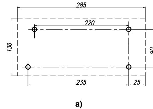
Рис.П7. Установочные размеры приборов ВЭРС-ПК(8,4,2)-02 ТРИО.
