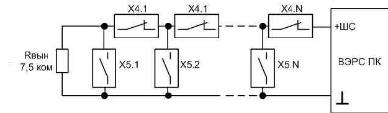
Рис.П6. Схема включения охранных извещателей.
