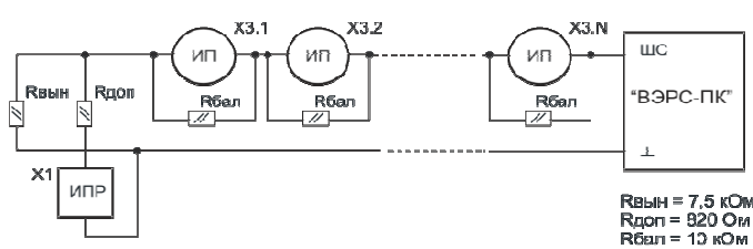
Рис.П4. Схемы включения ШС с несколькими тепловыми извещателями (типа ИП-105) и сработкой по двум извещателям (с перезапросом).
