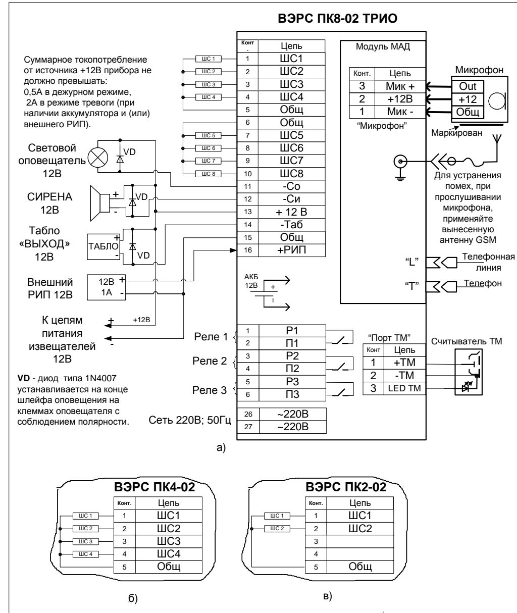
Рис.П2. Схемы внешних соединений приборов ВЭРС-ПК(8,4,2)-02 ТРИО.
