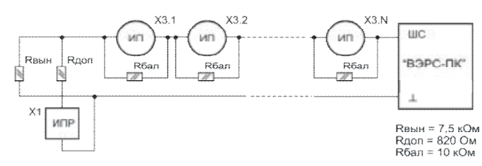
Рис.П4. Схемы включения ШС с несколькими тепловыми извещателями (типа ИП-105) и сработкой по двум извещателям (с перезапросом).
