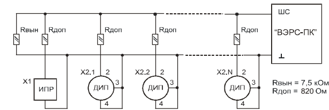
Рис.3. Схемы включения ШС типа ШННС и ШПНС с несколькими дымовыми извещателями (типа ИП212) и срабаткой по одному извещателю (с перезапросом).
