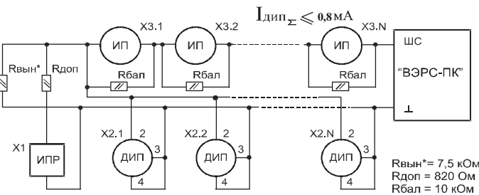
Рис.5. Комбинированная схема включения ШС типа ШННС со срабаткой по одному извещателю (с перезапросом).
