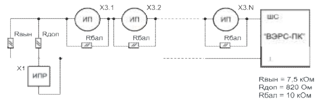
Рис.4. Схемы включения ШС типа ШННС с несколькими тепловыми извещателями (типа ИП-105) и срабаткой по двум извещателям (с перезапросом).
