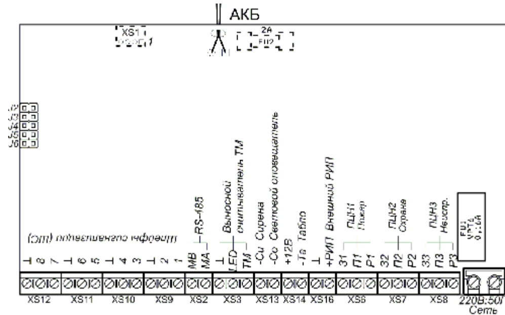
Рисунок А3. Вид на клеммы и разъемы для внешних подключений ВЭРС-ПК(8,4,2) Версия 3.1.
