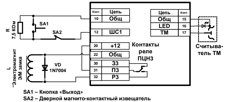
Рисунок Б7. Схема организации Точки доступа.
