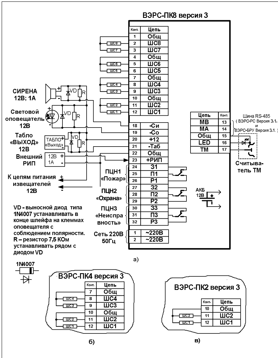
Рисунок.Б1. Схемы внешних соединений приборов ВЭРС-ПК(8,4,2) версия 3.1.
