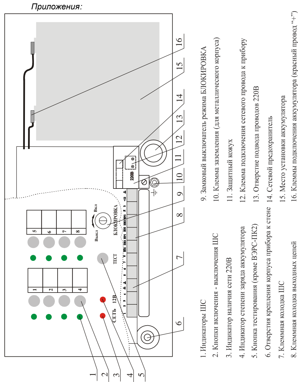
Рис. 1. Внешний вид и устройство приборов «ВЭРС-ПК2», «ПК4», «ПК8»
