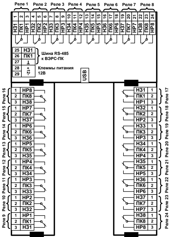
Рисунок А3. Схема внешних соединений ВЭРС-БРУ.
