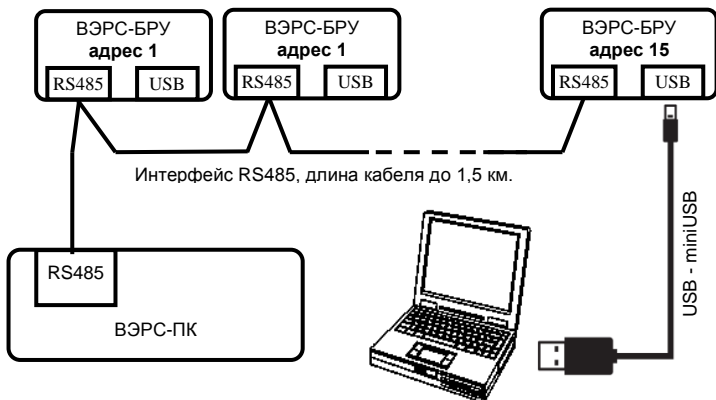
Рисунок А4. Структурная схема связи приборов ВЭРС-БРУ с ВЭРС-ПК(2,4,8,16,24) Версия 3.1.
