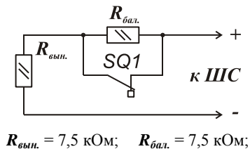
Рис. 2. Схема подключения датчиков с нормально замкнутыми контактами.
