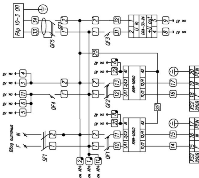
Рисунок 1А. Схема внутренних соединений шкафа.
